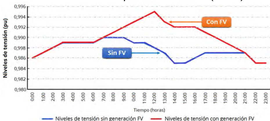
Gráfico III.5.15 Nivel de tensión de la fase r para la estación de verano (día hábil)
