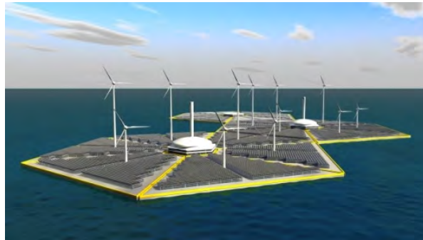
Figura III.4.9 Imagen de una energy island
