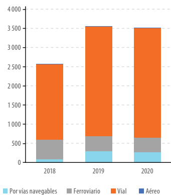
Indicador 9.1.2 Volumen de carga, por medio de transporte, 2018-2020 (En miles de millones de toneladas por kilómetro)
