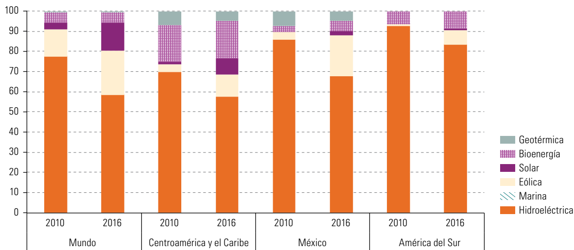
Capacidad instalada de generación eléctrica a partir de fuentes renovables en regiones seleccionadas, por tecnología, 2010 y 2016 (En porcentajes)
