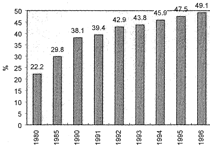
Gráfico 12 HONDURAS: INDICE DE ELECTRIFICACIÓN
