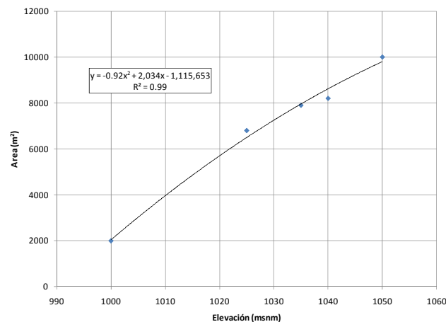
GRÁFICO 4.5 EMBALSE CENTRAL DE LA HIDROELÉCTRICA FORTUNA: CURVA DE ÁREA-ELEVACIÓN
