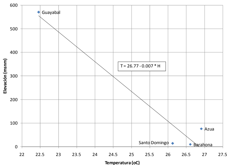
GRÁFICO 5.6 EMBALSE DE SABANA YEGUA: MODELO DE TEMPERATURA
