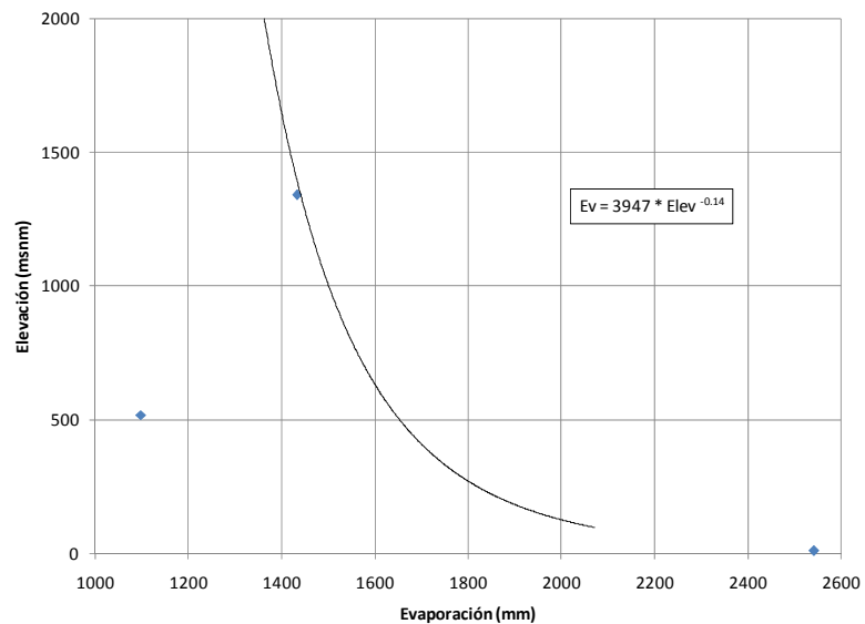
GRÁFICO 5.3 EMBALSE DE SABANA YEGUA: RELACIÓN ENTRE LA EVAPORACIÓN Y LA ELEVACIÓN
