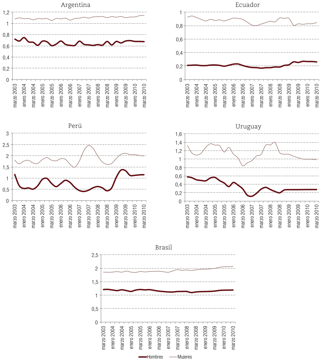
Gráfico 2 Valores estimados de \lambda_h, \lambda_m (sesgo de selección)
