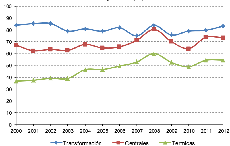
Gráfico 16 Eficiencia del sector transformación (En porcentajes)
