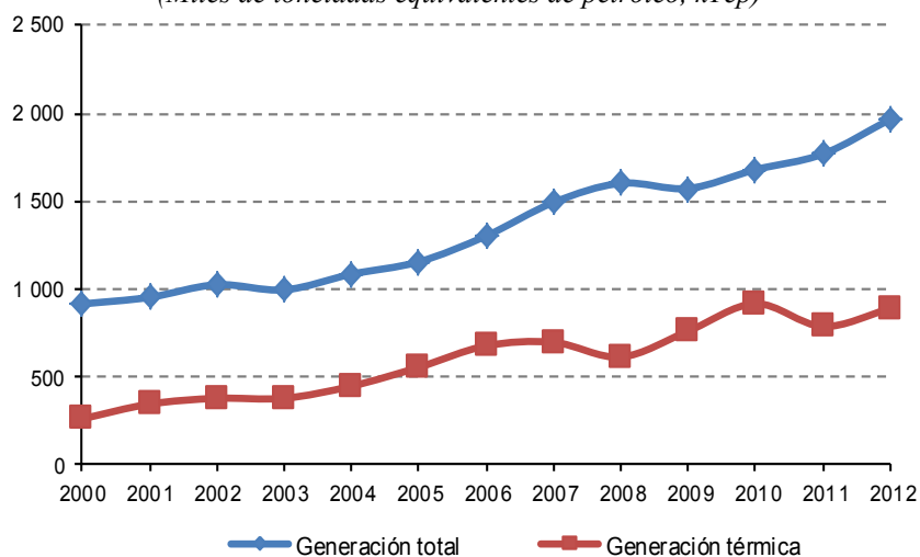
Gráfico 15 Generación eléctrica (Miles de toneladas equivalentes de petróleo, kTep)
