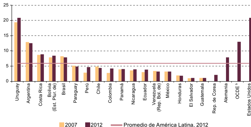
Gráfico IV.2 Densidad de la red vial total, 2007 y 2012 a (En kilómetros por cada 1.000 habitantes)
