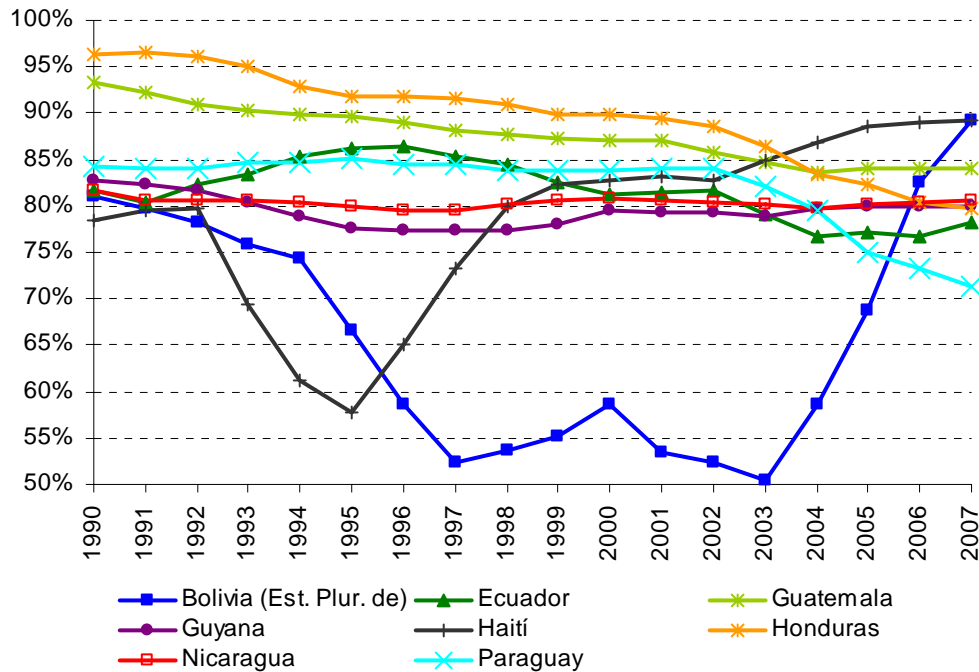
GRÁFICO A1.5 EFICIENCIA DEL ABASTECIMIENTO ENERGÉTICO (Países con PIB per cápita entre menor a 2.000 US$2000 / hab.)
