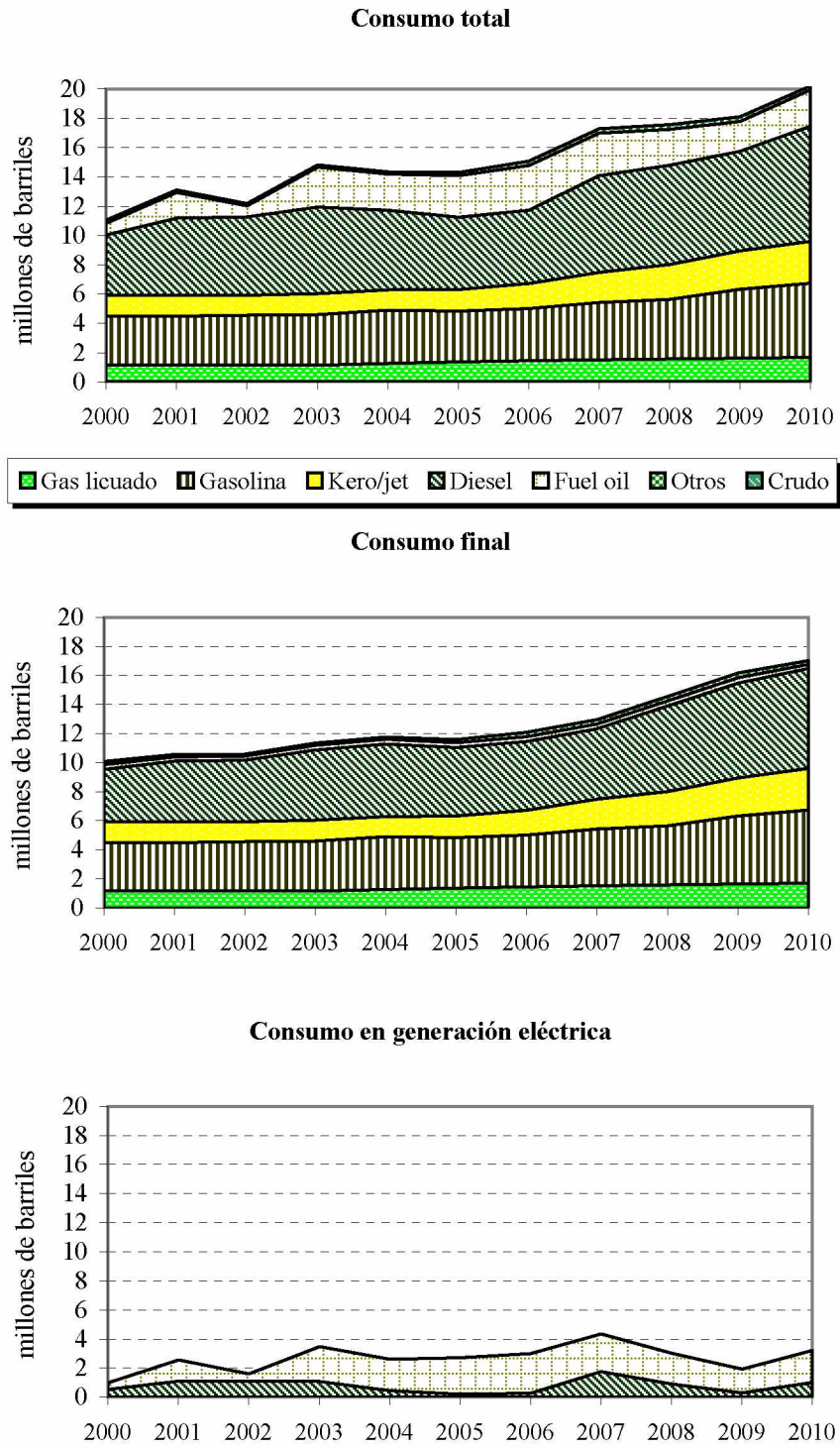
GRÁFICO 15 PANAMÁ: CONSUMO DE DERIVADOS DEL PETRÓLEO, 2000-2010
