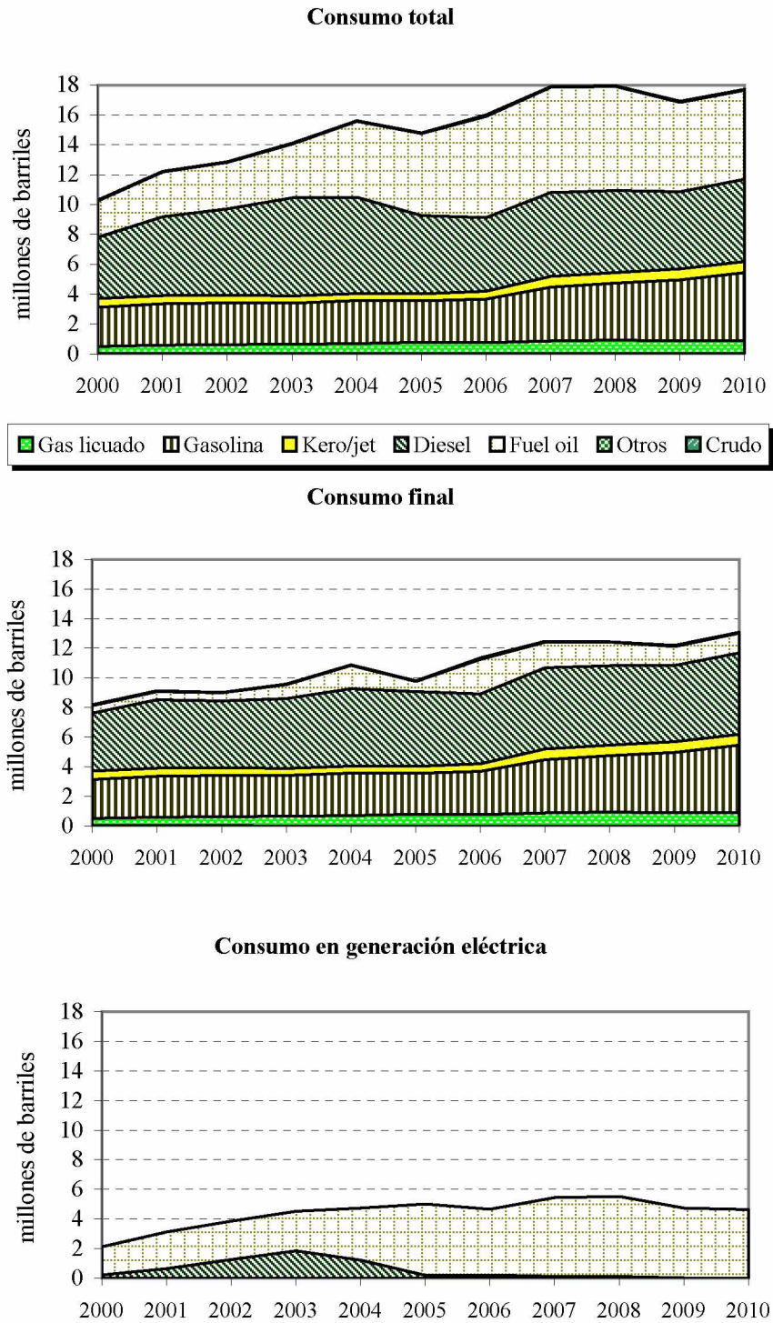
GRÁFICO 13 HONDURAS: CONSUMO DE DERIVADOS DEL PETRÓLEO, 2000-2010
