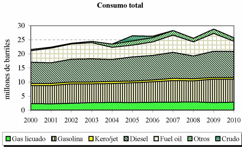
GRÁFICO 12 GUATEMALA: CONSUMO DE DERIVADOS DEL PETRÓLEO, 2000-2010
