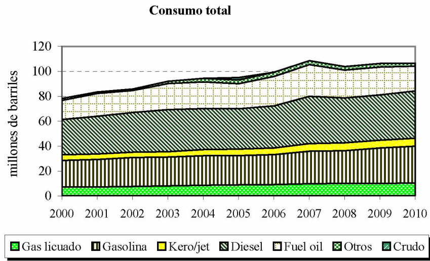
GRÁFICO 9 CENTROAMÉRICA: CONSUMO DE DERIVADOS DEL PETRÓLEO, 2000-2010
