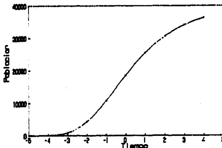
Gráfico 5 EVOLUCION DE LA POBLACION SEGUN LA FUNCION DE GOMPERTZ
