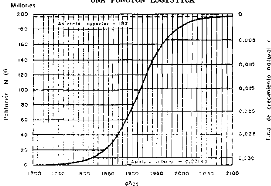
Gráfico 4 EVOLUCION DE LA POBLACION SEGUN UNA FUNCION LOGISTICA
