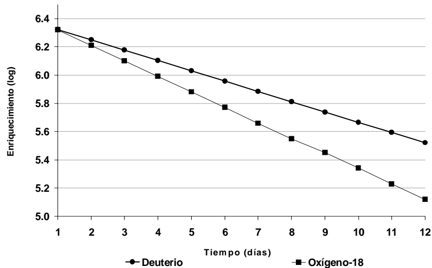
GRÁFICO 1 DIAGRAMA DE LA DESAPARICIÓN DE LOS ISÓTOPOS DE ^2\text{H} Y ^{18}\text{O} LUEGO DE LA INGESTA DE AGUA DOBLEMENTE MARCADA
