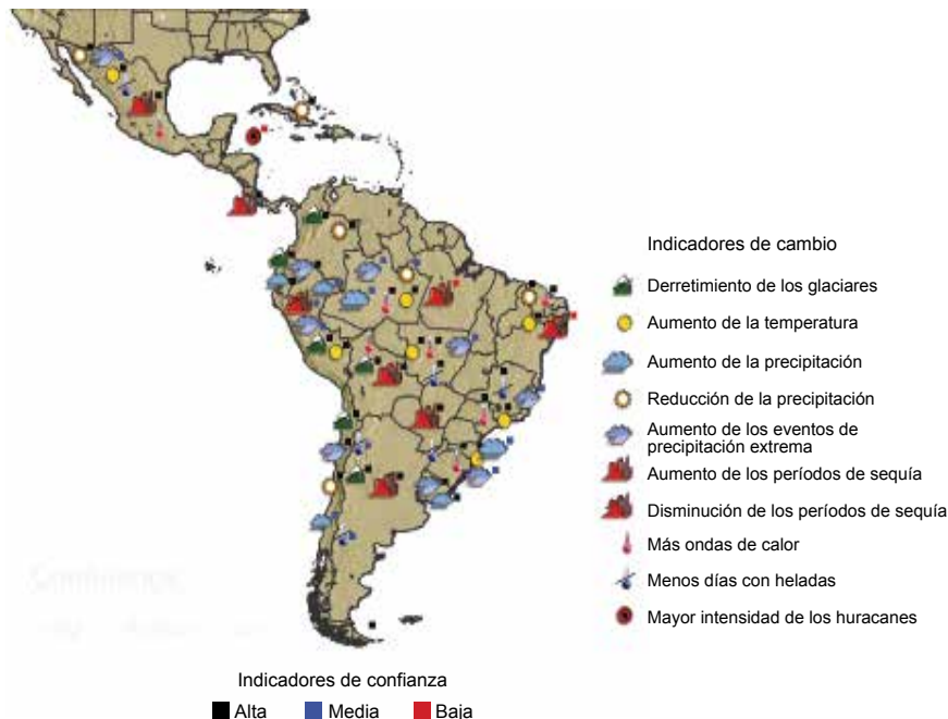
Mapa 1.1 AMÉRICA LATINA Y EL CARIBE: SÍNTESIS DE LOS PATRONES DE CAMBIO CLIMÁTICO PROYECTADOS HASTA 2100 a
