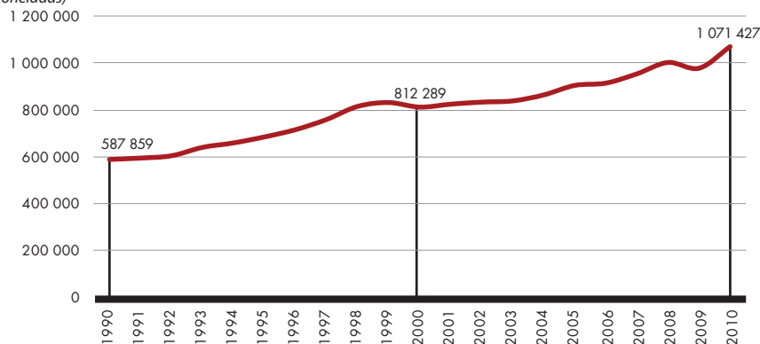
GRÁFICO IV.8. Unión de Naciones Suramericanas (UNASUR) (12 países): emisiones de dióxido de carbono (CO 2 ), 1990-2010
