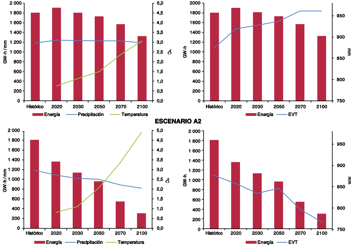
GRÁFICO 20 PLANTA CHIXOY: RESULTADOS DE SIMULACIONES, 2020 A 2100 ESCENARIO B2
