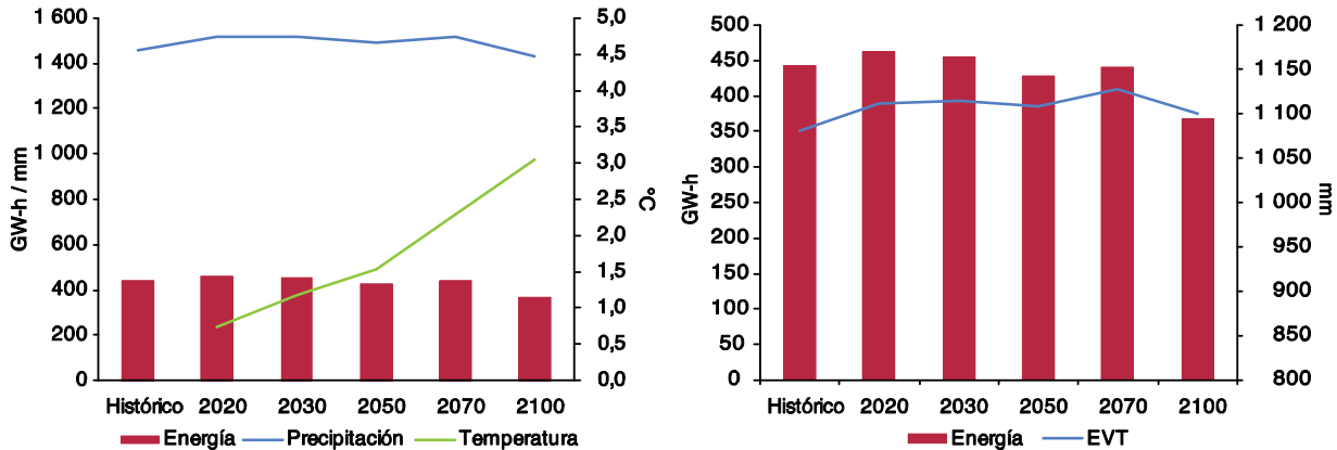
GRÁFICO 21 PLANTA CERRÓN GRANDE: RESULTADOS DE SIMULACIONES, 2020 A 2100 ESCENARIO B2
