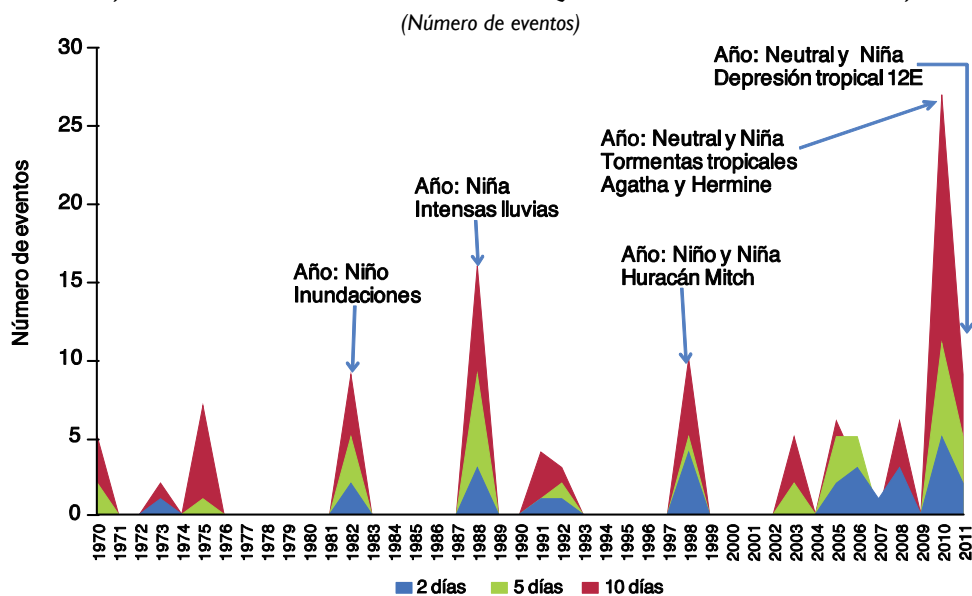
GRÁFICO 17 GUATEMALA, INSIVUMEH: NÚMERO DE EVENTOS QUE SOBREPASAN UMBRALES, 1970-2011
